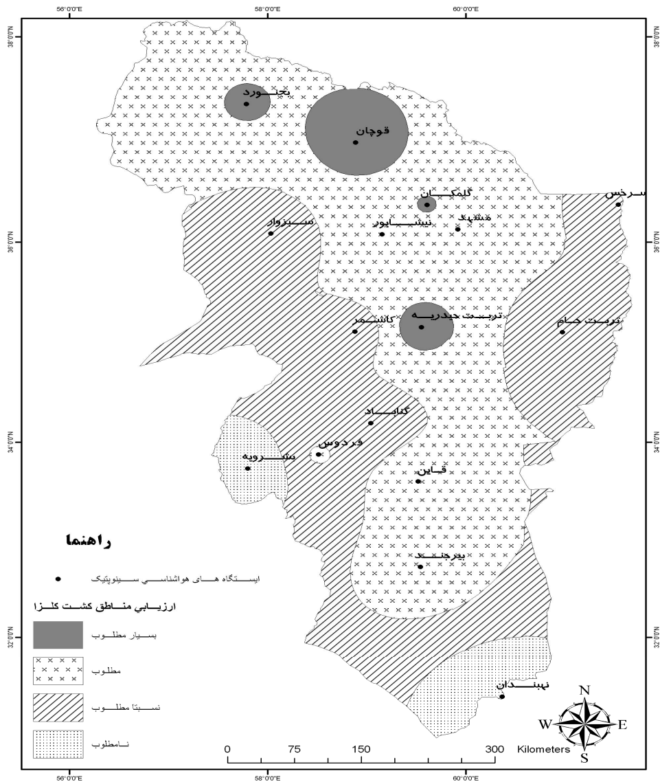
شکل ۱- نقشه توزیع جغرافیایی مناطق بهینه بندی کشت کلزا
