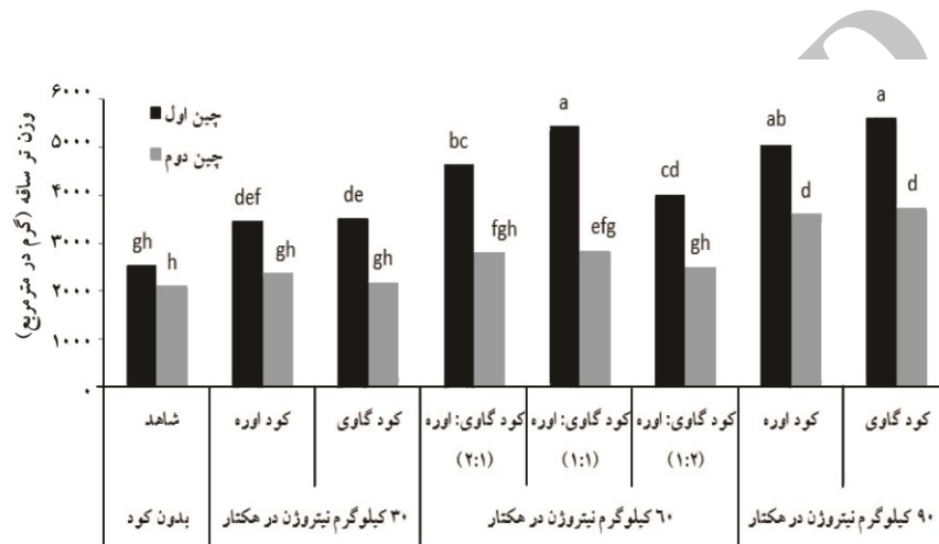
شکل ۵- اثر منابع و مقادیر مختلف کود نیتروژن بر مقدار وزن تر ساقه گیاه دارویی خرفه.
