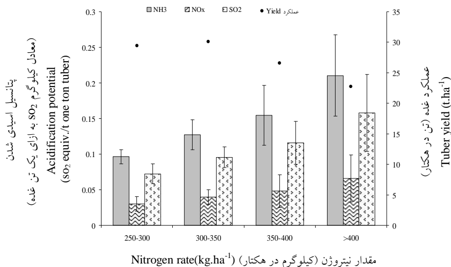
شکل ۴- پتانسیل اسیدی شدن یک واحد کارکردی نظام تولید سیب‌زمینی در سطوح مختلف کود نیتروژن.
