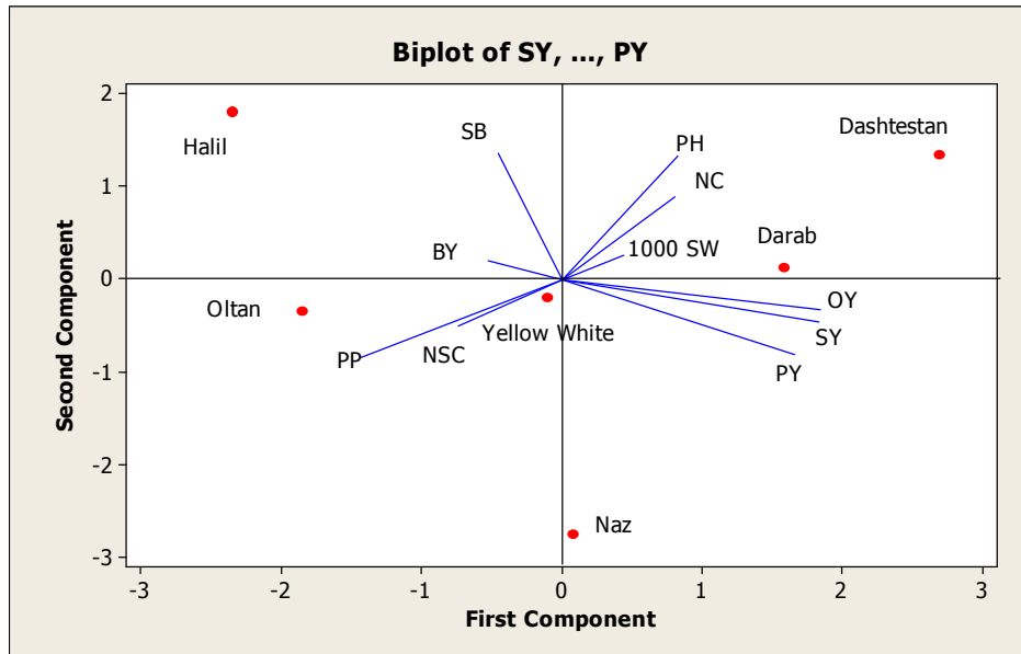
شکل ۲- نمودار دو بعدی صفات مورد بررسی در ۶ رقم کنجد براساس دو مؤلفه اول در شرایط تنش خشکی
