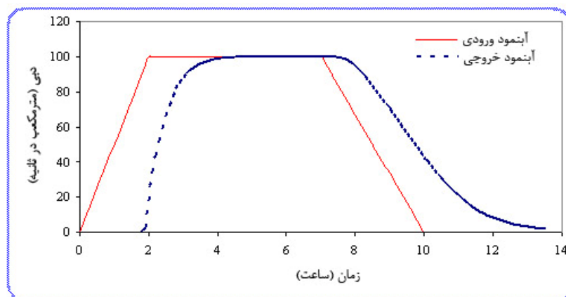
شکل (۲) - مشخصات آبنمود جریان یکنواخت و آبنمود خروجی روندیابی شده بوسیله مدل روندیابی دینامیکی
