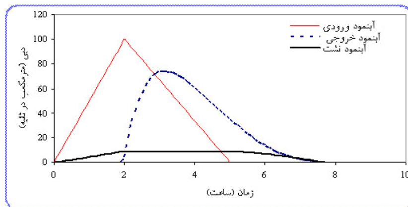
شکل (۳) - مشخصات آبنمود ورودی مثلثی، آبنمود خروجی و تلفات انتقال روندیابی شده بوسیله مدل روندیابی دینامیکی
