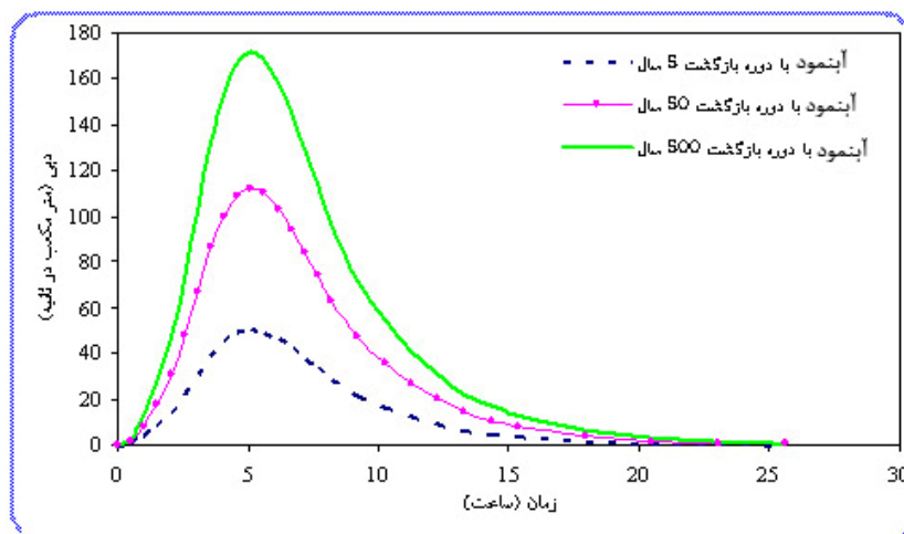
شکل (۶) - مشخصات آبنمودهای ورودی ۵، ۵۰ و ۵۰۰ ساله رودخانه زشک در محل ایستگاه سرآسیاب شاندیز
