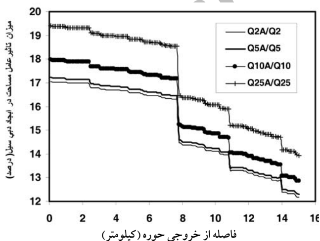
شکل ۶ - نمودارهای درصد تاثیر عامل مساحت در ایجاد دبی با دوره بازگشت های مختلف نسبت به فاصله از خروجی حوزه شمرد
