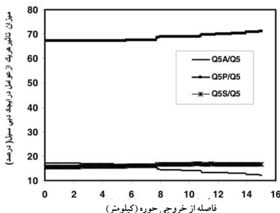
شکل ۱۰- نمودارهای درصد تأثیر هر یک از عوامل در ایجاد دبی با دوره بازگشت پنج ساله نسبت به فاصله از خروجی حوزه شمرود
