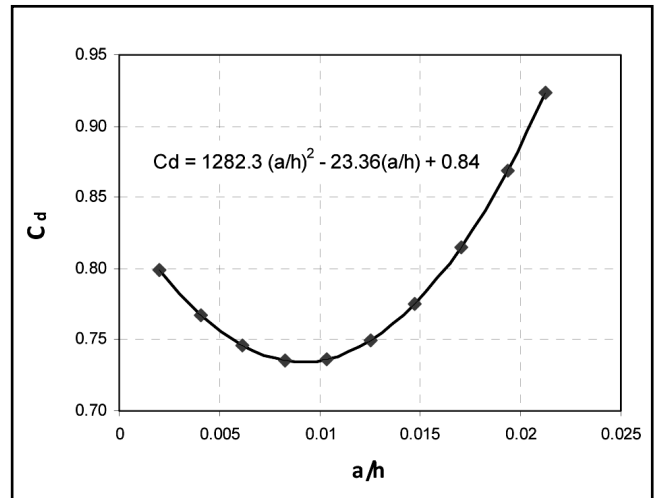
شکل ۱۳ - نمودار تغییرات ضریب آبگذری دریاچه
