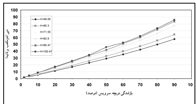
شکل ۷- نمودار تغییرات دبی در ترازهای مختلف به ازای بازشدگی های مختلف دریچه سرویس (در ۱۰۰ درصد بازگشایی دریچه اضطراری)
