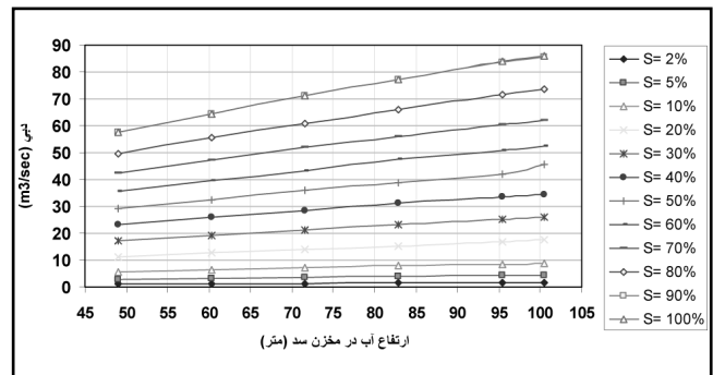
شکل ۱۱ - نمودار تغییرات دبی - تراز - بازشدگی دریاچه سرویس (در ۱۰۰ درصد بازشدگی دریاچه اضطرابی)
