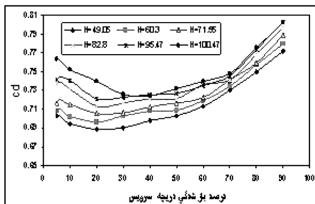
شکل ۹ - منحنی تغییرات ضریب آبگذری دریچه سرویس
