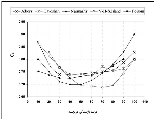
شکل ۱۴ - مقایسه بین منحنی ضریب آبگذری سد نرماشیر با سایر پژوهش‌های انجام شده
