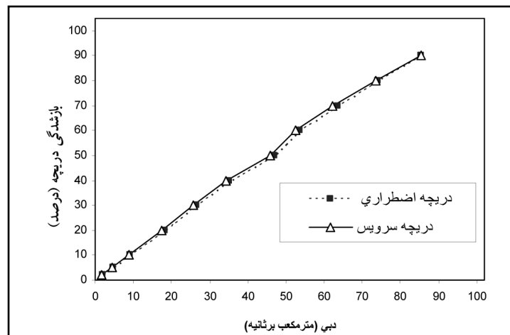
شکل ۶- منحنی تغییرات آنگذری دریچه ها در بازشدگی های مختلف
