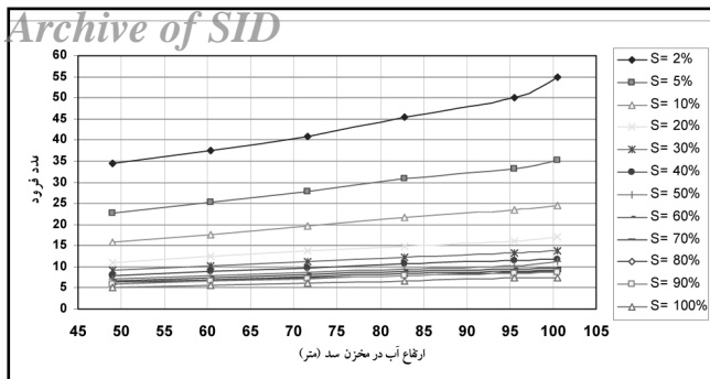
شکل ۱۲ - نمودار تغییرات عدد Fr در تراز و بازشدگی های مختلف دریاچه سرویس (در ۱۰۰ درصد بازشدگی دریاچه اضطرابی)
