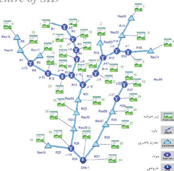
شکل (۲) - حوزه آبخیز تجریش در محیط HEC-HMS
