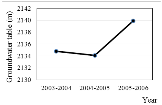
شکل ۴- هیدروگراف واحد آبخوان طی سالهای ۸۵-۱۳۸۲
