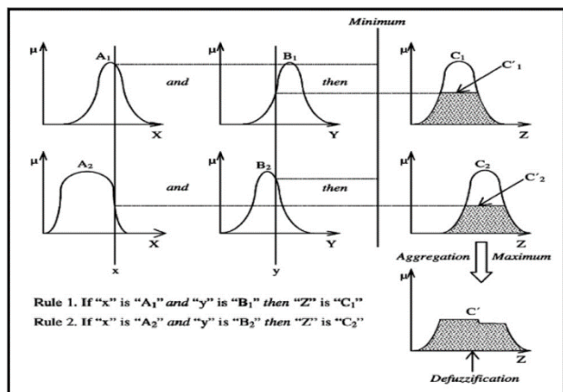
شکل ۳- سیستم استنتاج فازی ممدانی [۱۵]
