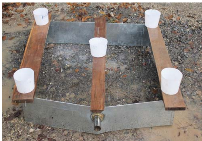
شکل ۳- چیدمان جمع‌آوری‌کننده‌ها برای تعیین شدت و ضریب یکنواختی باران
