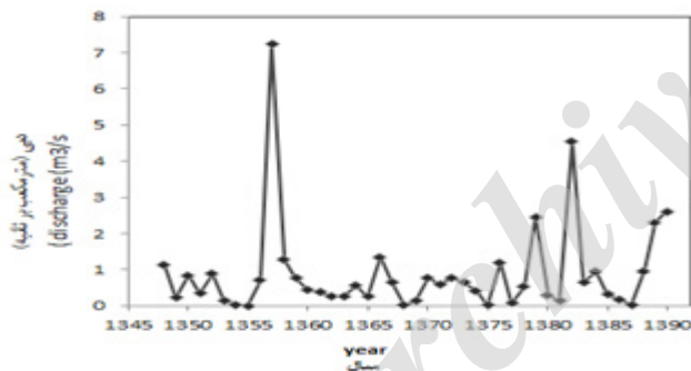
شکل ۱۲- نمودار آبدهی شهریور ماه Figure 12. September discharge Chart
