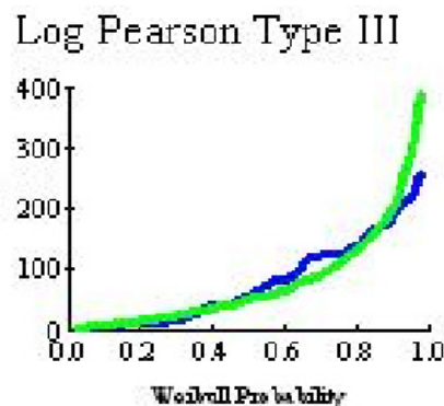
شکل ۱۴- توزیع آماری در ایستگاه هیدرومتری تمر Figure 14. Statistical distribution in Tamar Hydrometric station
