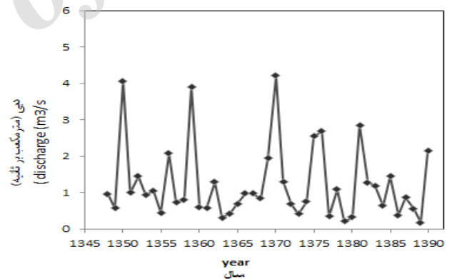
شکل ۹- نمودار آبدهی خرداد ماه Figure 9- June discharge Chart
