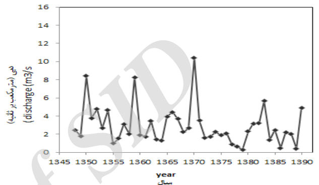
شکل ۸- نمودار آبدهی اردیبهشت ماه Figure 8. May discharge Chart
