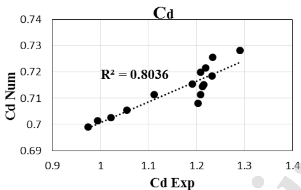
شکل ۴- رابطه ضریب دبی آزمایشگاهی و عددی
