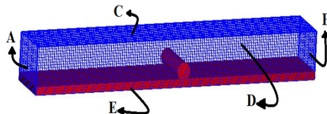
شکل ۳- تعریف شرایط مرزی در مدل مورد نظر
