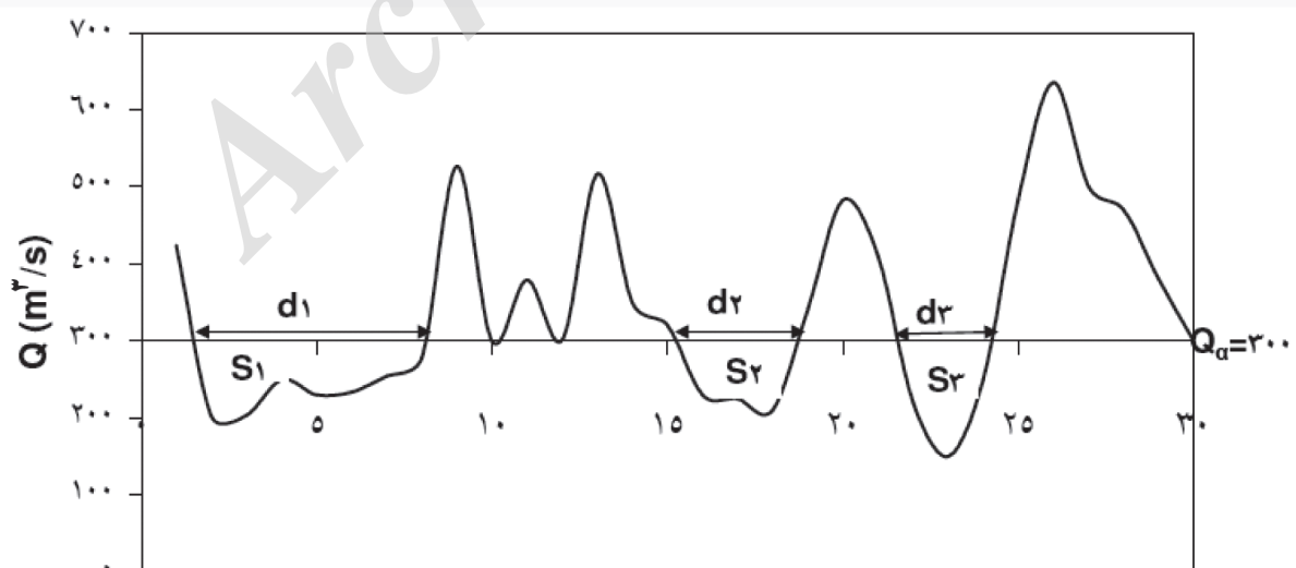
شکل ۲- بر اساس روش حد آستانه ثابت S_i حجم کمبود خشکسالی و d_i مولفه‌های تداوم
