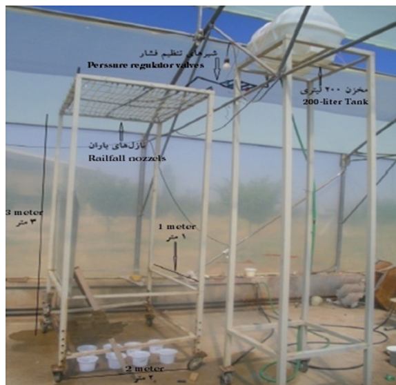
شکل ۱- دستگاه باران‌ساز طراحی شده در گلخانه علوم خاک دانشگاه زنجان و استفاده شده در این پژوهش
