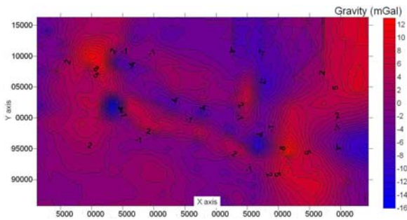
کل ۷.۷. بی‌هنجاری باقی‌مانده با استفاده از برازش چند جمله‌ای درجه سه.
