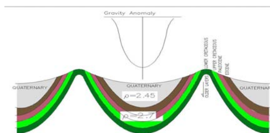
شکل ۱۱. مدل فرضی زمین شناسی منطقه شکل ۱۲ گرانی باقی مانده اطراف حوزه رسوبی.
