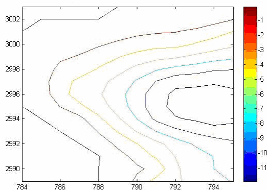
شکل ۱۲. گرانی مشاهده شده در اطراف حوزه رسوبی.
