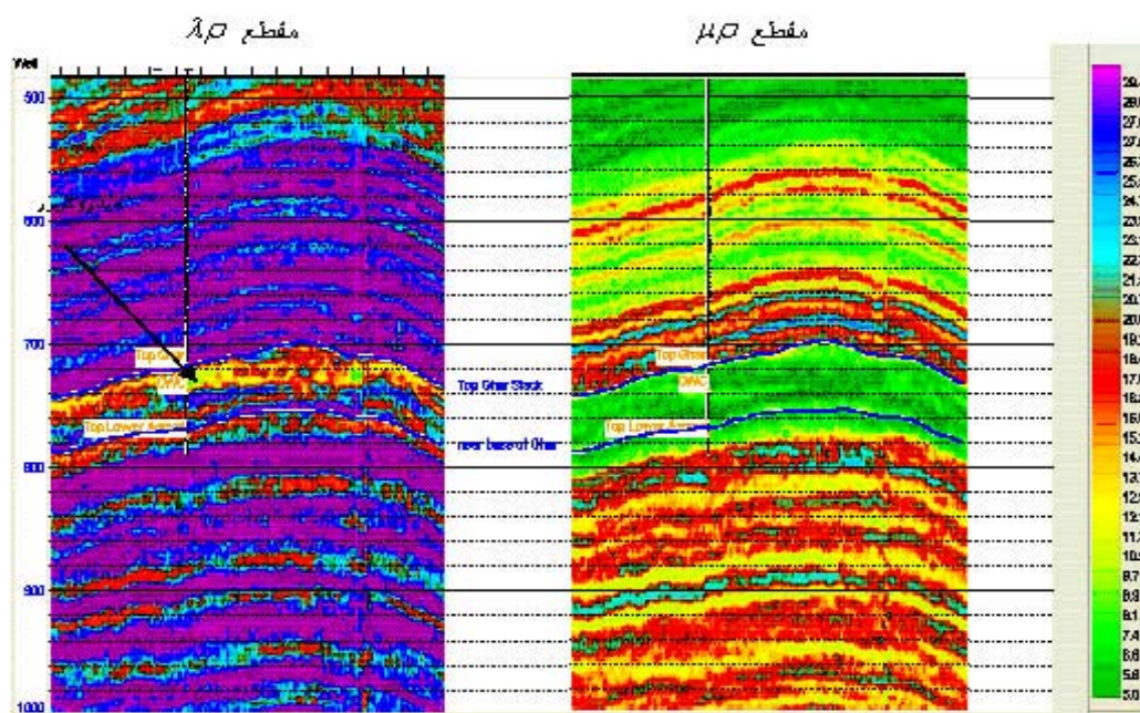
شکل ۶. مقاطع \lambda\rho و \mu\rho ، کاهش غیر معمول در مقطع \lambda\rho نشان‌دهنده حضور هیدروکربور است همان‌طور که ملاحظه می‌شود مقطع \mu\rho در قسمت ماسه‌سنگ مخزن مقدار کمتری نسبت به لایه‌های کربناته و انیدریتی بالا و پایینی مخزن دارد. مقیاس رنگی، تغییرات پارامترهای لامه را نشان می‌دهد.
