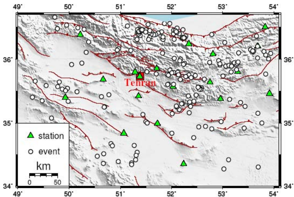
شکل ۱. پراکندگی ۱۷۹ زلزله مورد بررسی (دایره‌های سفید) و ایستگاه‌های لرزه‌نگاری (مثلث‌های سبز) در ناحیه تهران. همه زلزله‌های با بزرگی بیش از ۳ و گاز آزیموتی کمتر از ۲۵۰ که در سال‌های ۱۹۹۶ تا ۲۰۰۴ روی داده‌اند در این تحقیق در نظر گرفته شده‌اند. خطوط پیوسته، محل گسل‌های فعال منطقه را نشان می‌دهند (حسامی و همکاران، ۲۰۰۳).
