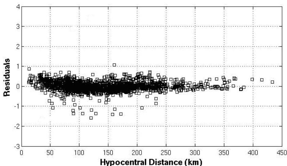
شکل ۵. مقدار باقی‌مانده بزرگی M_1 برحسب فاصله. یک انحراف از مقدار متوسط صفر در فواصل کمتر از ۴۰ کیلومتر (محل پیکان عمودی) دیده می‌شود.
