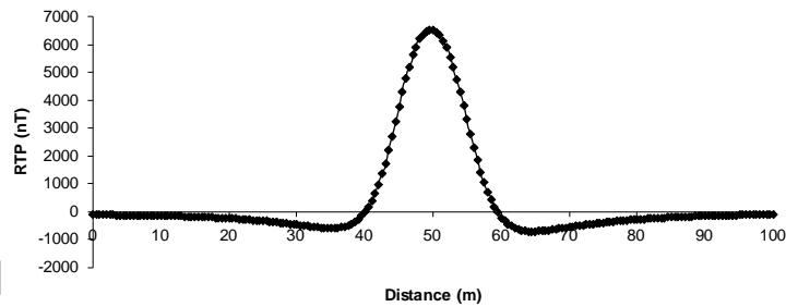
شکل ۲. منحنی بی‌هنجاری بازمانده مدل اول در طول نیم‌رخ AA
