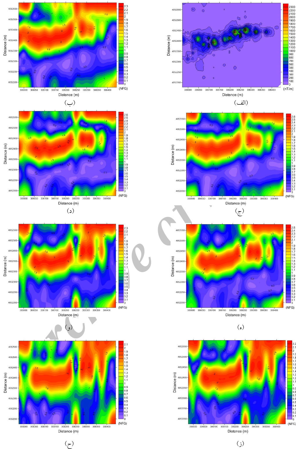
شکل ۱۵. نقشه سیگنال تحلیلی و NFG برای عمق‌های متفاوت، (الف) نقشه سیگنال تحلیلی، (ب) نقشه NFG سه‌بعدی در عمق صفر متر، (ج) نقشه NFG سه‌بعدی در عمق ۲۰ متر و (د) نقشه NFG سه‌بعدی در عمق ۴۰ متر، (ه) نقشه NFG سه‌بعدی در عمق ۶۰ متر، (و) نقشه NFG سه‌بعدی در عمق ۸۰ متر، (ز) نقشه NFG سه‌بعدی در عمق ۱۰۰ متر و (ح) نقشه NFG سه‌بعدی در عمق ۱۲۰ متر.
