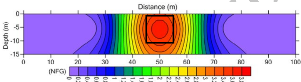
شکل ۹. نقشه NFG حاصل از مدل سوم.
