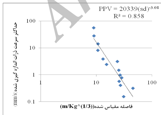
شکل ۳. نمودار حداکثر سرعت ذرات نسبت به فاصله مقیاس شده در سد گتوند علیا.
