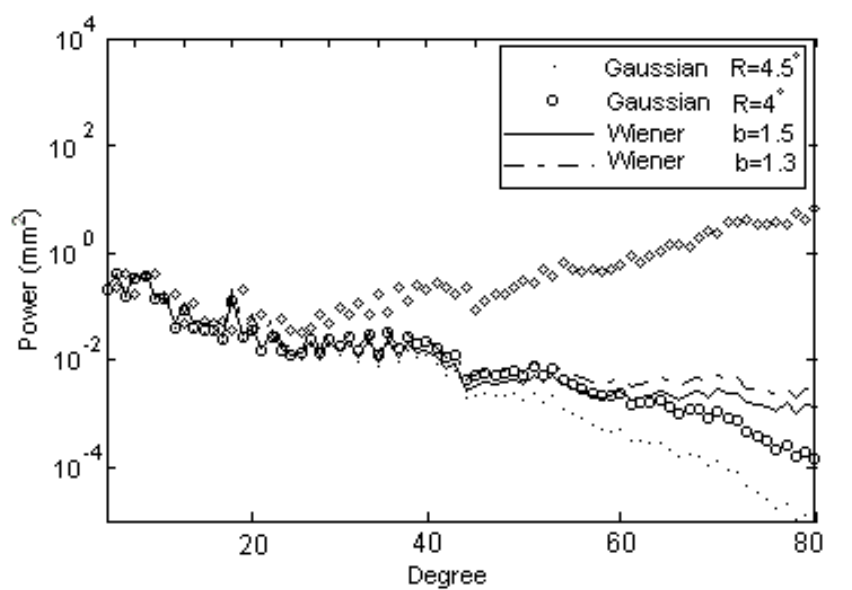
شکل ۸. اعمال ضرایب وزن فیلتر بهینه وینر و گاوسی روی توان طیفی مدل ماهیانه برحسب ارتفاع ژئوئید برای ماه پنجم از سال ۱۳۸۷ (مربع‌های توخالی).
