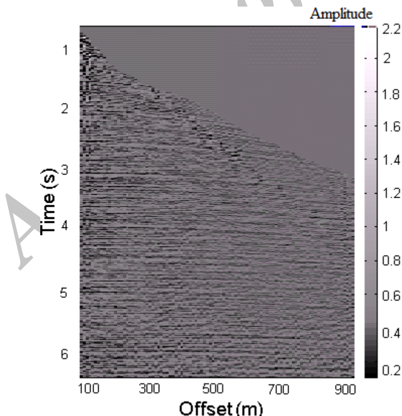
شکل ۹. ورداشت نقطه میانی مشترک واقعی در یکی از مناطق لرزه‌نگاری جنوب کشور.
