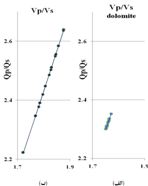
شکل ۷. مقایسه نمودارهای چاه III: (الف) V_p/V_s (از رابطه کاستاگنا) برحسب Q_p/Q_s و (ب) V_p/V_s (از DSI) برحسب Q_p/Q_s .
