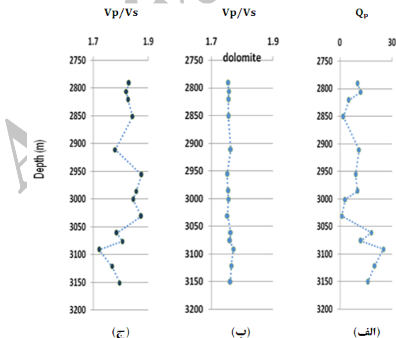
شکل ۵. مقایسه نمودارهای چاه III برحسب عمق: (الف) Q_p ، (ب) V_P/V_S برای دولومیت (از رابطه کاستاگنا) و (ج) V_P/V_S از نگاره DSI.
