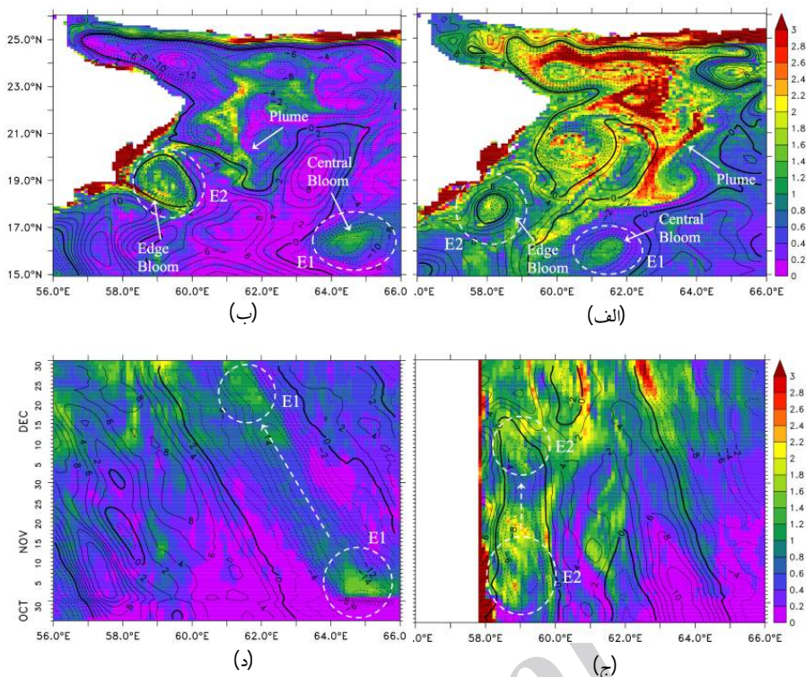
شکل 8. غلظت سبزینه سطحی و تراز سطح آب در مدل‌های CM2.6 و miniBLING در ماه‌های نوامبر و دسامبر در سالی که تقابل بین شکوفایی و پیچک در بخش جنوبی منطقه مشاهده شده است در (الف) ماه نوامبر، (ب) 28 دسامبر، (ج) طی نوامبر و دسامبر در 16 درجه شمالی و (د) طی نوامبر و دسامبر در 19 درجه شمالی.
