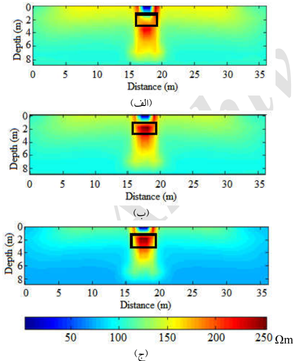
شکل ۱۲. نتایج تصویرسازی با روش کمترین مربعات میرا برای مقادیر مقاومت ویژه ظاهری مدل شکل ۲ حاصل شده از آرایه ونر- شلومبرژه با مقادیر پارامتر \lambda (الف) ۰/۵ و (ب) ۵ و (ج) ۵۰. موقعیت توده مقاومتی مدفون با مستطیل سیاه‌رنگ روی شکل‌ها مشخص شده است.
