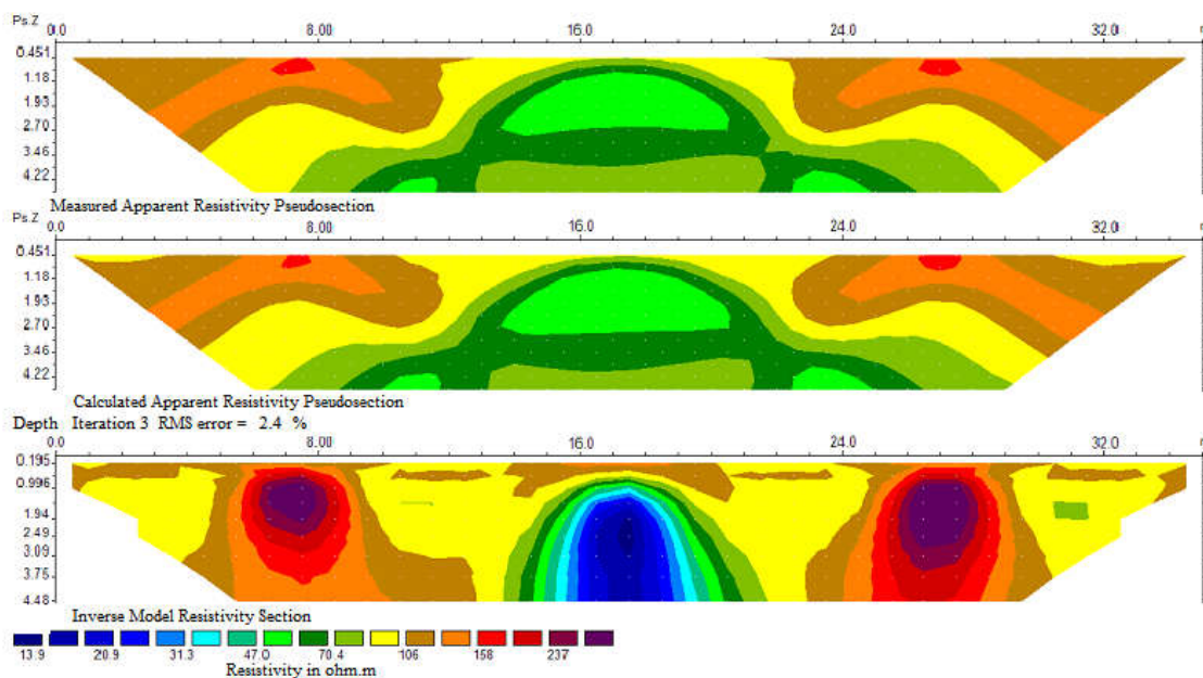
شکل ۲۰. مدل مقاومت ویژه زیرسطحی حاصل از وارون‌سازی استاندارد کمترین مربعات (مقطع پایینی) داده مقاومت ویژه ظاهری اندازه‌گیری شده برای مدل شکل ۱۶ با آرایه دوقطبی - دوقطبی (شبه مقطع بالایی) با استفاده از نرم‌افزار RES2DINV. شبه مقطع میانی مقدار مقاومت ویژه ظاهری محاسبه شده از وارون‌سازی می‌باشد.
