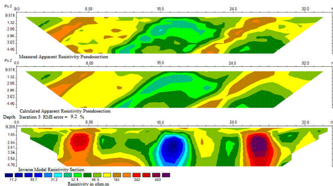
شکل ۲۶. مدل مقاومت ویژه زیرسطحی حاصل از وارون‌سازی استاندارد کمترین مربعات (مقطع پایینی) داده مقاومت ویژه ظاهری اندازه‌گیری شده برای مدل شکل ۱۶ با آرایه قطبی-دوقطبی (شبه مقطع بالایی) با ۱۰٪ نوفه تصادفی اضافه شده به وسیله نرم‌افزار RES2DINV. شبه مقطع میانی مقدار مقاومت ویژه ظاهری محاسبه شده از وارون‌سازی می‌باشد.
