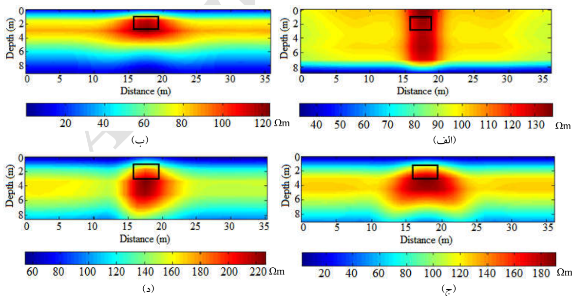
شکل ۵. مدل‌های پس‌بینی (تصویرسازی وارون) به دست آمده با استفاده از B^T بر اساس معادله (۶) برای آرایه‌های (الف) ونر-شلمبرژه، (ب) ونر، (ج) دوقطبی-دوقطبی و (د) قطبی-دوقطبی. موقعیت توده مقاومتی مدفون با مستطیل سیاه‌رنگ روی شکل‌ها مشخص شده است.
