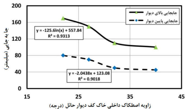
شکل ۶. تأثیر زاویه اصطکاک داخلی خاک کف دیوار حائل بر جابه‌جایی لرزه‌ای دیوار.
