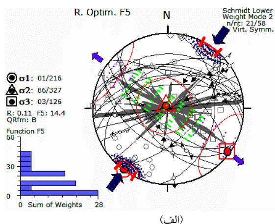
شکل ۱۳. (الف) تانسور تنش حل شده با استفاده از برگردان داده‌های سازوکار کانونی زمین‌لرزه‌ها. نمودار سمت چپ پایین توزیع گاوسی دارد و بیانگر زاویه ناهمخوانی بین جهت بیشینه لغزش حل شده و واقعی است، (ب) نمودار گل‌سرخ‌ی روندهای انتخاب شده براساس زاویه لغزش. به‌عنوان صفحه گسلی، اکثر صفحات روند شرقی- غربی نشان می‌دهند.
