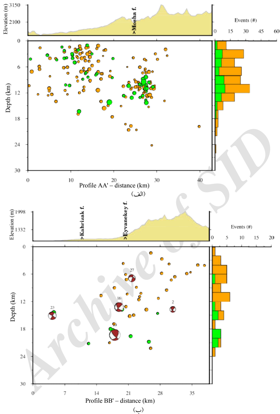
شکل ۴. (الف) مقطع عمقی AA' که توزیع عمقی زمین‌لرزه‌ها را عمود بر روند گسل مشا نشان می‌دهد. (ب) مقطع عمقی BB' که توزیع عمقی زمین‌لرزه‌ها را عمود بر بخش شمالی گسل ایوانکی (پارچین) نشان می‌دهد. رنگ‌ها مربوط به دو کلاس A و C است.
