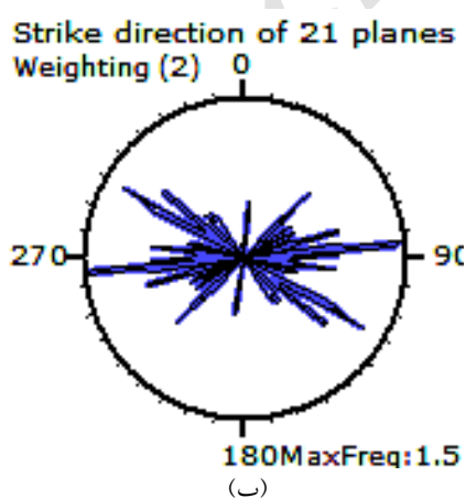
شکل ۱۳. (الف) تانسور تنش حل شده با استفاده از برگردان داده‌های سازوکار کانونی زمین‌لرزه‌ها. نمودار سمت چپ پایین توزیع گاوسی دارد و بیانگر زاویه ناهمخوانی بین جهت بیشینه لغزش حل شده و واقعی است، (ب) نمودار گل‌سرخ‌ی روندهای انتخاب شده براساس زاویه لغزش. به‌عنوان صفحه گسلی، اکثر صفحات روند شرقی- غربی نشان می‌دهند.
