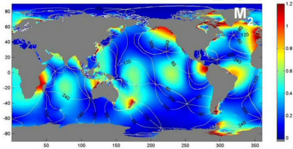
شکل ۲. مؤلفه کشتندی M_2 در مدل جهانی کشتند TPXO
