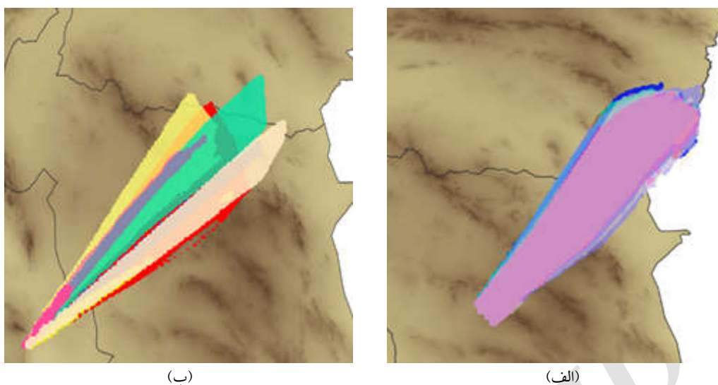
شکل ۱۳. تفاوت شبیه‌سازی محدوده پخش مواد باروری با مدل پاشندگی HYSPLIT حاصل از اجرای هشت ترکیب‌بندی از پارامترسازی‌های فیزیکی در مدل هواشناسی WRF. شکل (الف) مربوط به پرواز شماره ۳۱ در تاریخ ۲ فوریه ۲۰۱۷ و شکل (ب) مربوط به پرواز شماره ۳۸ در تاریخ ۱۷ فوریه ۲۰۱۷ در منطقه شرق کشور، در استان‌های خراسان جنوبی و رضوی است.
