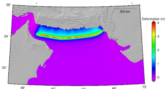
شکل ۲. میدان دگرشکلی محاسبه شده (برحسب متر) برای سناریوی با بزرگای ۹/۱
