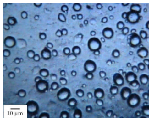
شکل ۵. اثر به‌جای‌مانده قطرک‌های آبرسد روی لامل در زیر میکروسکوپ نوری.
