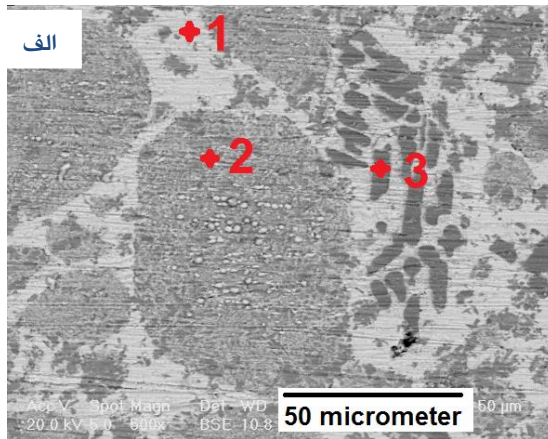
شکل ۲: الف) آنالیز نقطه‌ای پراش انرژی پرتوی ایکس از فازهای مختلف آمالگام. ب) تصویر نمونه‌ی دیسکی تهیه شده
