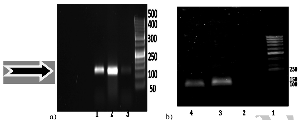
شکل ۲- تکثیر ژن IL-1 \alpha
