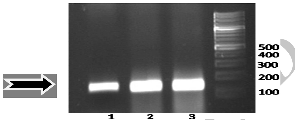
شکل ۱- تکثیر ژن GAPDH
