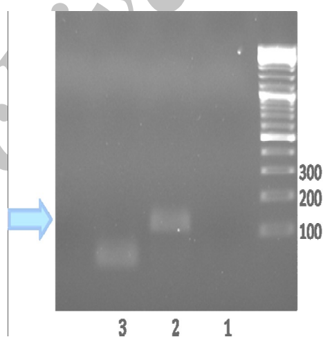
شکل ۳- تکثیر ژن IL-1 \beta
