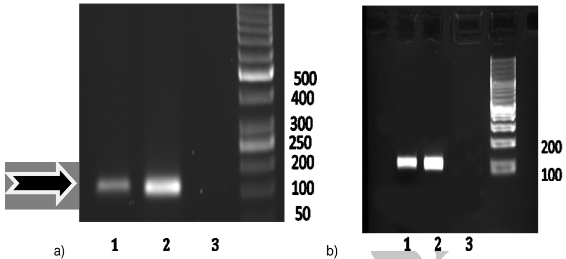
شکل ۴- تکثیر ژن IL-8
