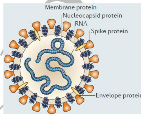
شکل ۱: ساختار ویروس کوروناویروس MERS (۲۶)
