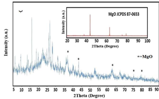
شکل ۱. الگوی پراش اشعه ایکس زئولیت موردنیت بزرگ (الف) و نانوذرات منیزیم اکسید در ماتریس زئولیتی (ب)
