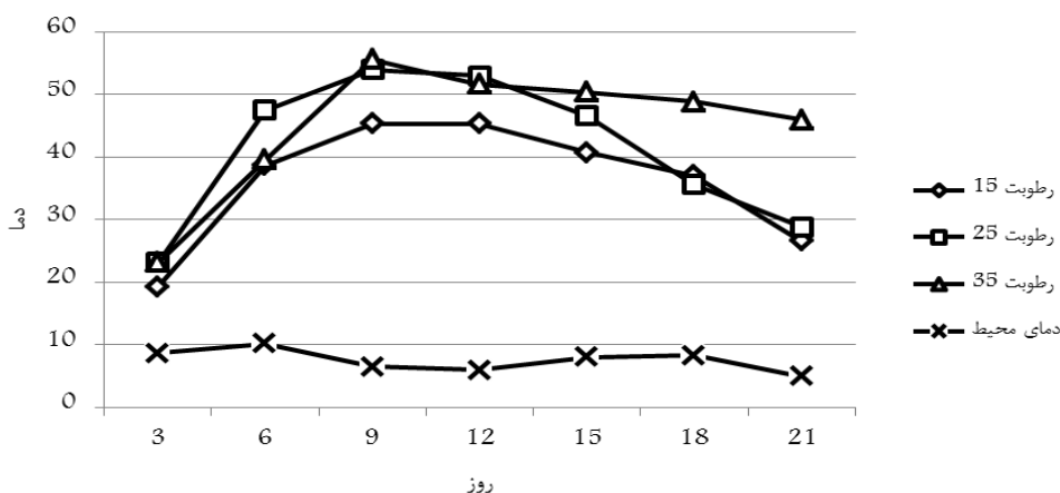
شکل ۳. نمودار اثر سطح رطوبت (درصد) بر دمای (درجه سلسیوس) بستر جوجه گوستی دپوشده در عمق ۶۰ سانتی متر
