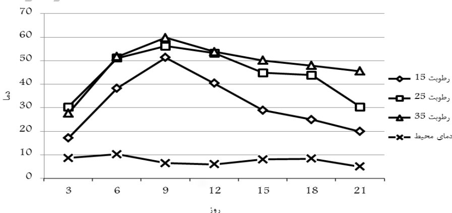
شکل ۲. نمودار اثر سطح رطوبت (درصد) بر دمای (درجه سلسیوس) بستر جوجه گوسشتی دپوشده در عمق ۳۰ سانتی‌متر
