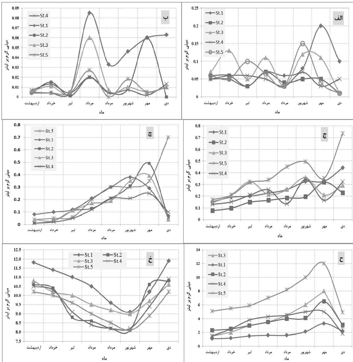
شکل ۲- نتایج متغیرهای اندازه‌گیری شده در طول دوره نمونه‌برداری و در ایستگاه‌های پنجگانه. الف- تغییرات میزان فسفات، ب- تغییرات میزان نیتريت، ج- تغییرات میزان نترات، چ- تغییرات میزان آمونیاک، ح- تغییرات میزان BOD 5 و خ- تغییرات میزان DO
