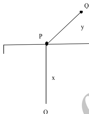
شکل ۲- روش نمونه برداری T-square: x بین نقطه o و نزدیک‌ترین فرد یعنی p و y بین فرد p و نزدیک‌ترین همسایه یعنی Q، در انتخاب افرادی که در همان طرف نیم صفحه مثل o قرار می‌گیرند، در نظر گرفته نمی‌شوند (Ludwig and Reynolds, 1988).
