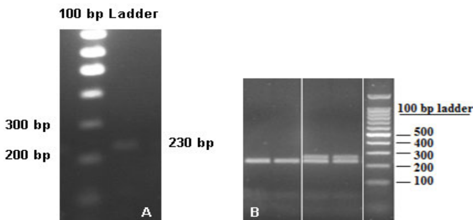
شکل ۲- ژل آگارز مربوط به برش آنزیمی قطعه ۲۸۰ جفت بازی ناحیه Na/K ATP-ase. تصویر (A): باند ۲۳۰ جفت بازی تولید شده از نمونه‌های آرتمیای طشک تصویر (B): ژل رفرنس گرفته شده از Manaffar et al. (2011). الگوی برش دو باندهی مربوط به آرتمیای پارتنوژن و الگوی تک باندهی نشانگر آرتمیای دو جنسی می باشد.
