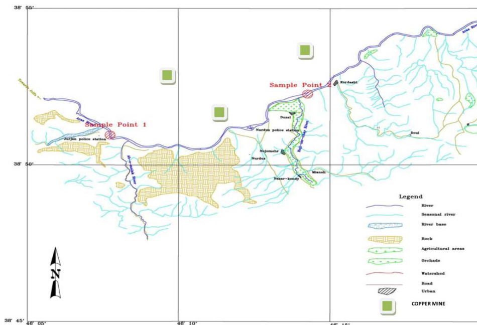
شکل ۲. ایستگاه‌های نمونه‌برداری
