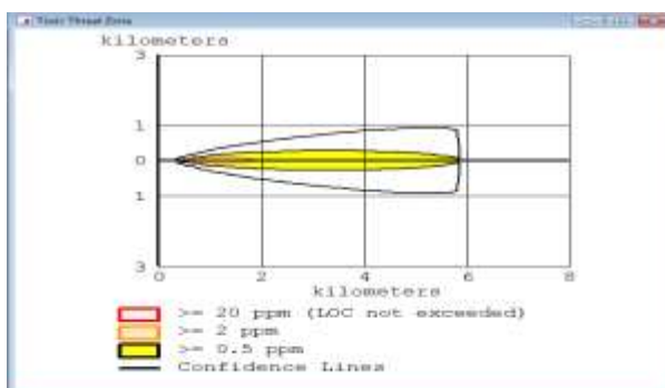
شکل ۱۴. مدلسازی پراکنش آلاینده‌ها در نرم‌افزار ALOHA
