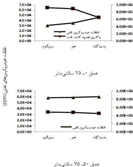
شکل ۲. تغییرات غلظت هیدروکربن‌های نفتی و تعداد باکتری نفت‌خوار در اعماق مختلف خاک
