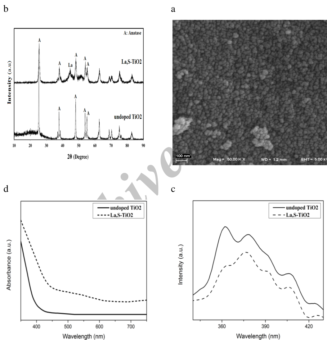
شکل شماره ۴: مشخصه‌یابی نانوفتوکاتالیست \text{TiO}_2/\text{S}/\text{La} : تست SEM، b: تست XRD، c: تست P.L، d: تست DRS
