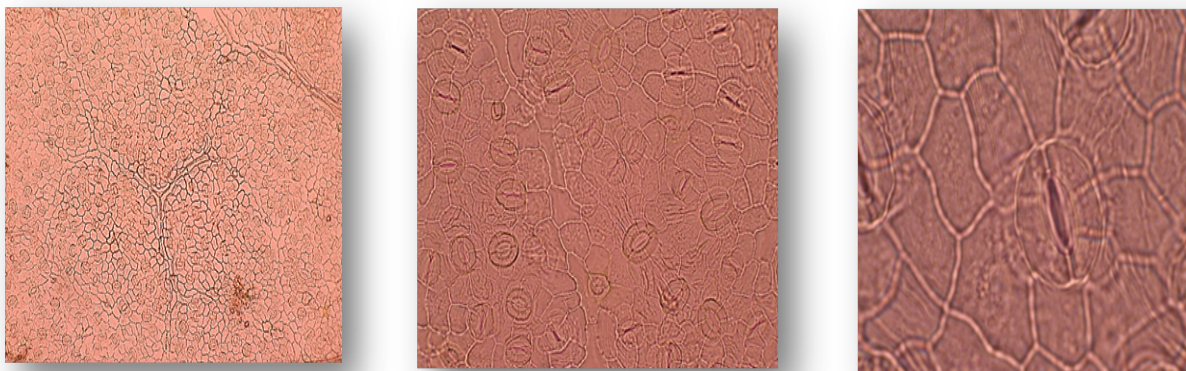
شکل ۴- مقطع طولی برگ و نمایش روزنه‌ها در سطح تحتانی برگ چنار (بزرگ‌نمایی از چپ به راست به ترتیب 10 \times ، 40 \times و 100 \times )
