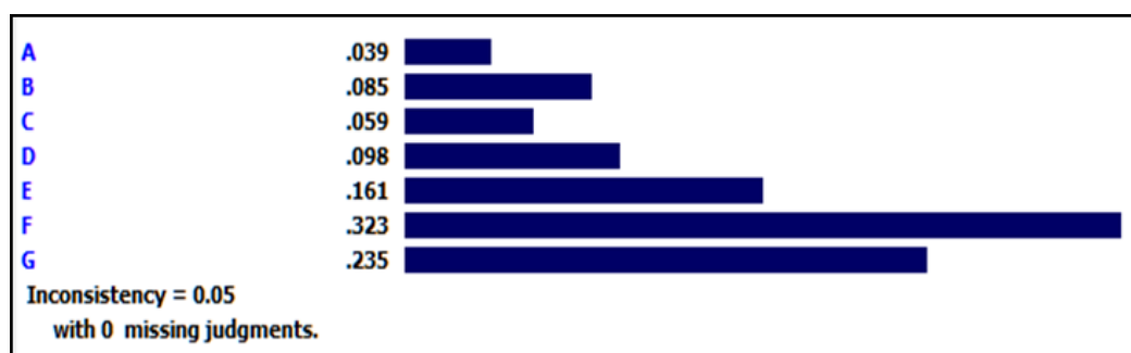
شکل ۵- میزان وزن و اهمیت هر یک از معیارهای مورد بررسی با استفاده از روش AHP
