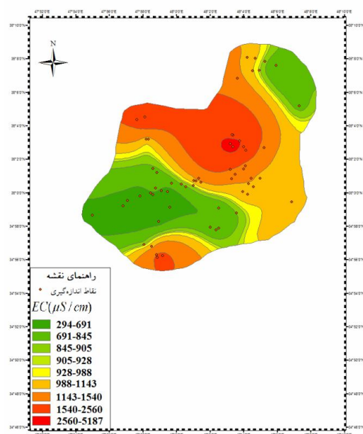
شکل (5) نقشه EC دشت چهاردولی قروه به روش کریجینگ
