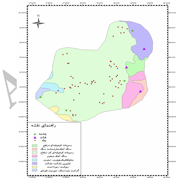
شکل 1- نقشه زمین‌شناسی دشت چهاردولی قروه به همراه نقاط نمونه برداری
