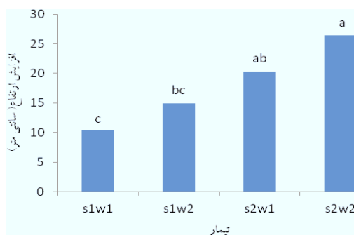
شکل ۱- اثر کیفیت آب آبیاری و سیستم آبیاری بر افزایش ارتفاع نهال زیتون
