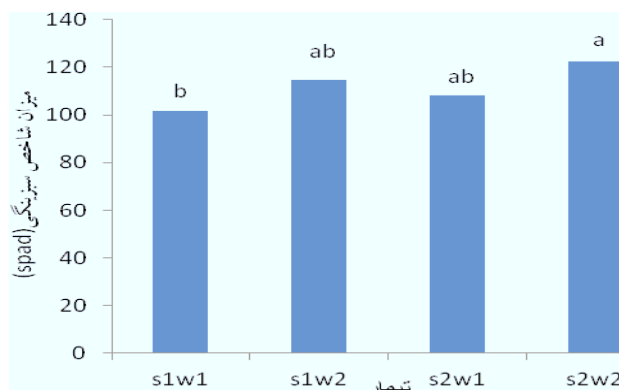
شکل ۲- اثر کیفیت آب آبیاری و سیستم آبیاری بر شاخص سبزینگی نهال زیتون ( s_1 =آبیاری سطحی، s_2 =آبیاری زیر سطحی، w_1 =آب معمولی، w_2 =آب فاضلاب تصفیه شده)
