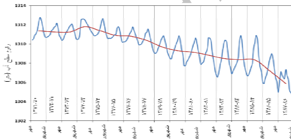
شکل ۴- هیدروگراف واحد آبخوان دشت میان‌در بند طی سال‌های ۱۳۷۱-۷۰ تا ۱۳۸۶-۸۷
