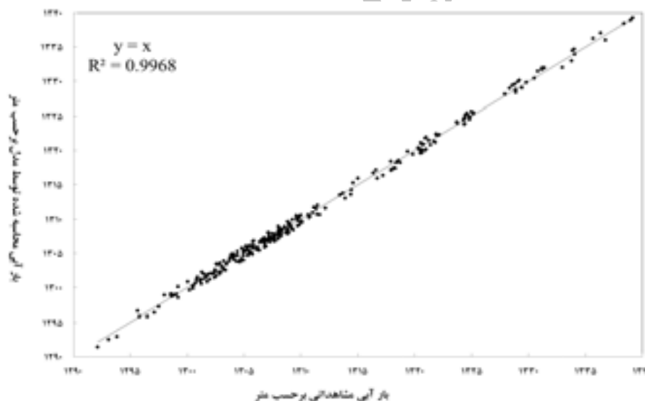
شکل ۷ - مقایسه سطح آب مشاهداتی و محاسباتی در پیژومترهای میان‌در بند در سال ۱۳۸۵
