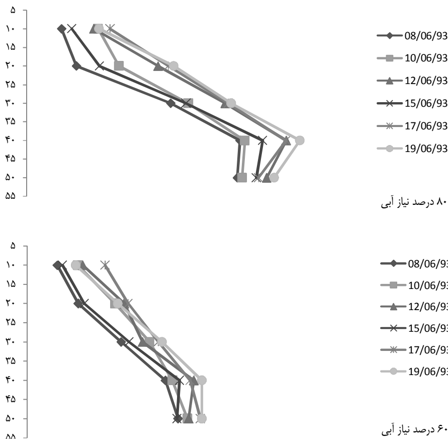
نمودار ۳- درصد رطوبت حجمی باقی مانده در عمق‌های مختلف و به ترتیب برای تیمارهای ۱۰۰، ۸۰ و ۶۰ درصد نیاز آبی
