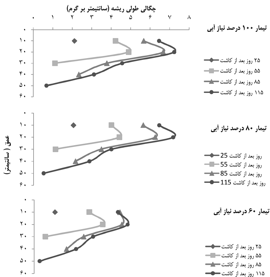
نمودار ۱- تراکم طولی ریشه در مقابل زمان در تیمارهای مختلف نیاز آبی
