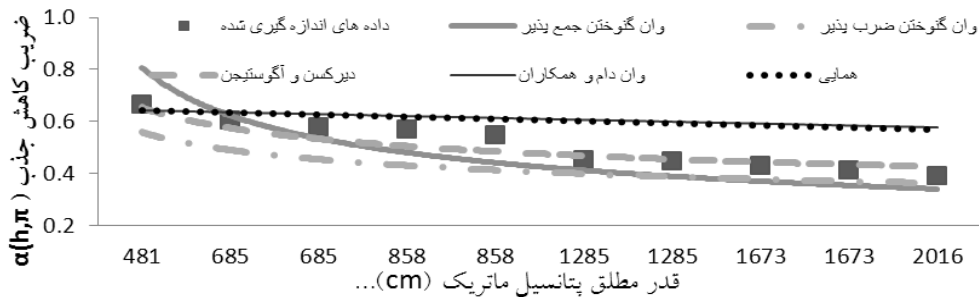
شکل ۱۰- برازش مدل‌های مختلف برداده‌های اندازه‌گیری شده حاصل از تیمار سطح شوری ۴/۵ dS/m و تخلیه ۶۰ درصد
